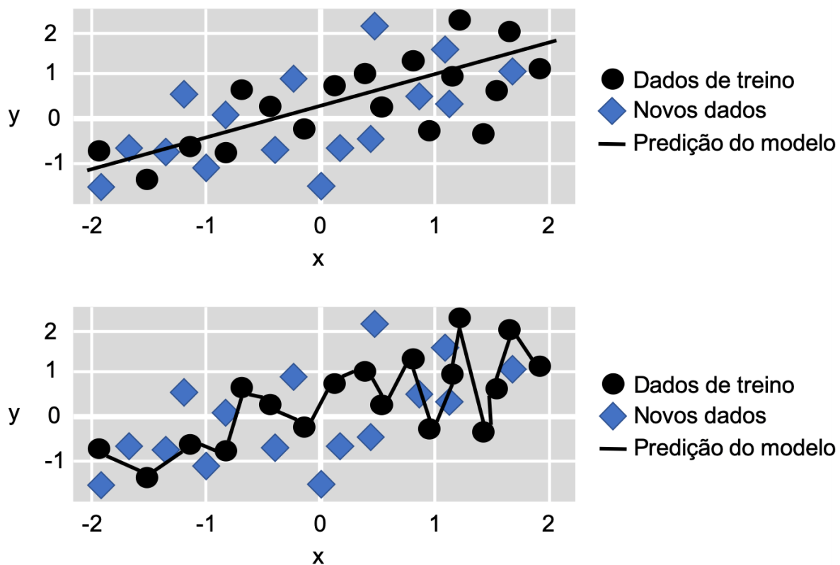
Figura 5.5: Exemplo de overfitting
